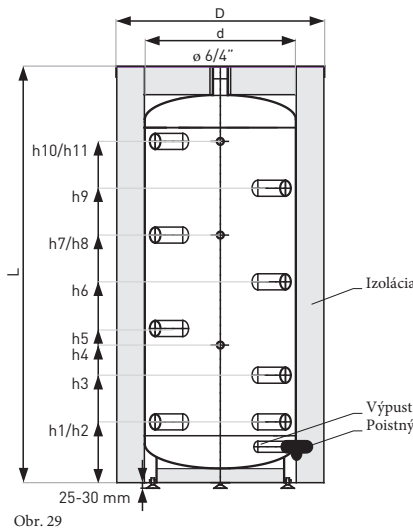
SCHÉMA AKUMULAČNEJ NÁDRŽE obj. 300-2000 l.
