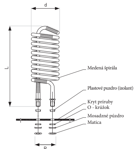
SCHÉMA MONTÁŽE medeného špirál. ohrievača v prírubu
