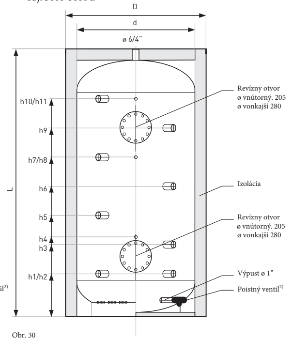
SCHÉMA AKUMULAČNEJ NÁDRŽE obj. 3000-5000 l.
