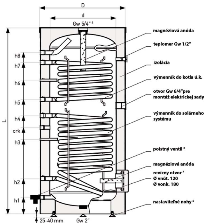
QUADROFLEX QFS 2P / 200 - 300 - 700 - 1000
